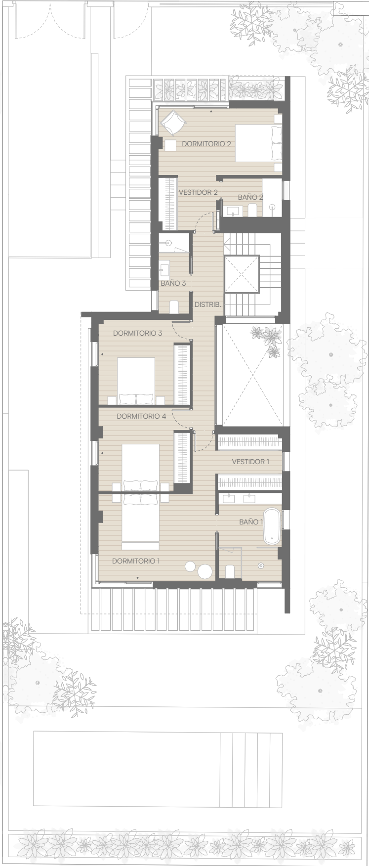
PLANTA PRIMERA
