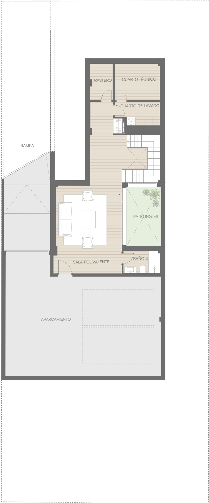
PLANTA SÓTANO
