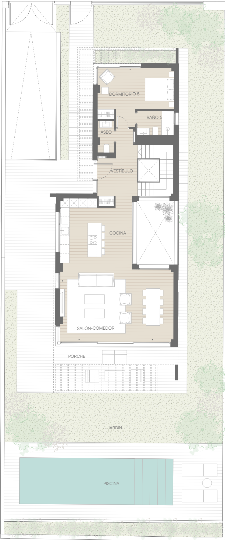
PLANTA BAJA
